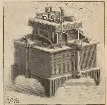
Fig. 2. - Transformador de la Sociedad de alumbrado eléctrico para la alimentación de las bujías Jablochhoff
